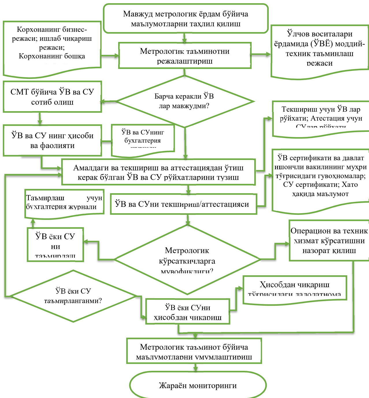
1-расм. Қурилиш материаллари ишлаб чиқариш корхонасини сифат менежменти тизими асосида “Назорат ва ҳисоблаш ускуналарини бошқариш” жараёнининг алгоритми
